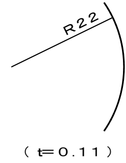
A-A' 鋼材断面図
